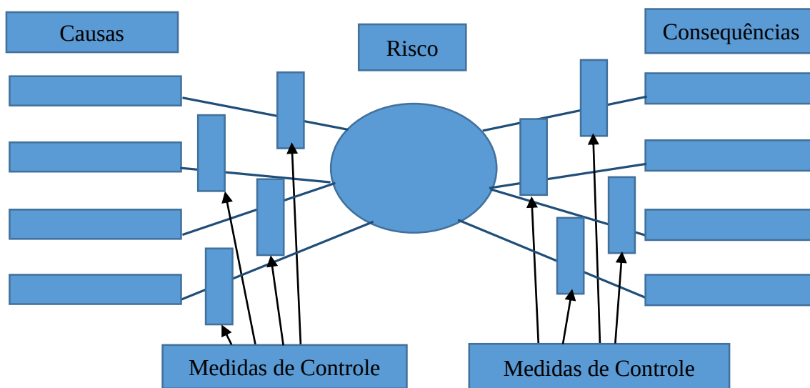
Figura 3: Técnica Bow-tie.
