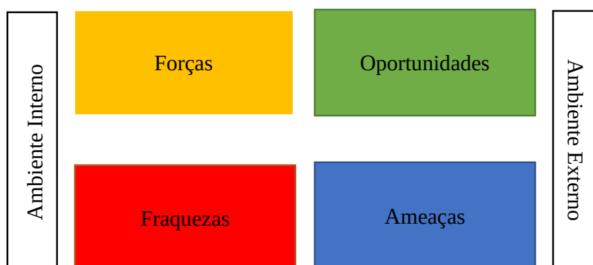
Figura 4: Ferramenta SWOT.
