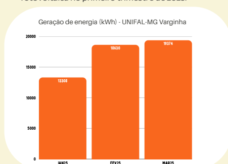
Gráfico de geração de energia da usina fotovoltaica no primeiro trimestre de 2025.
