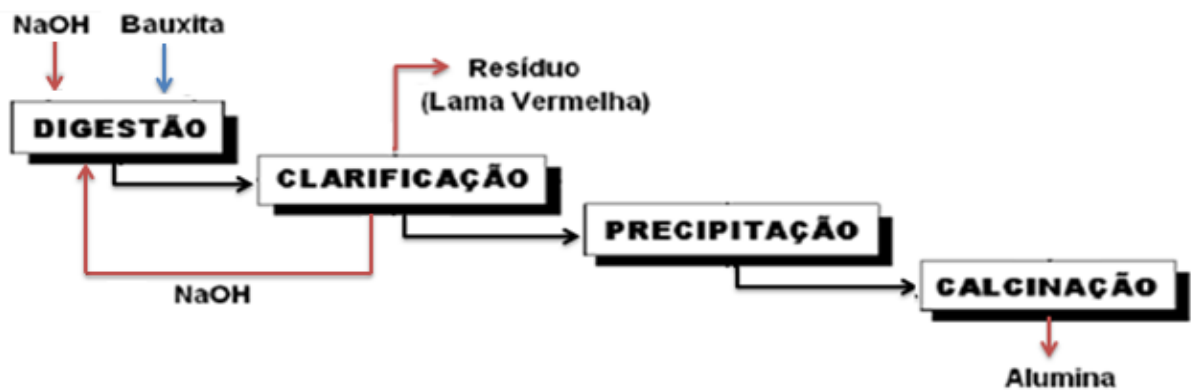
Figura 1 - Fluxograma das etapas do processamento da bauxita para formação de alumina no Processo Bayer.
